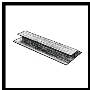
H профиль из алюминия для стеновой панели из ДПК 32x70x3600 мм
